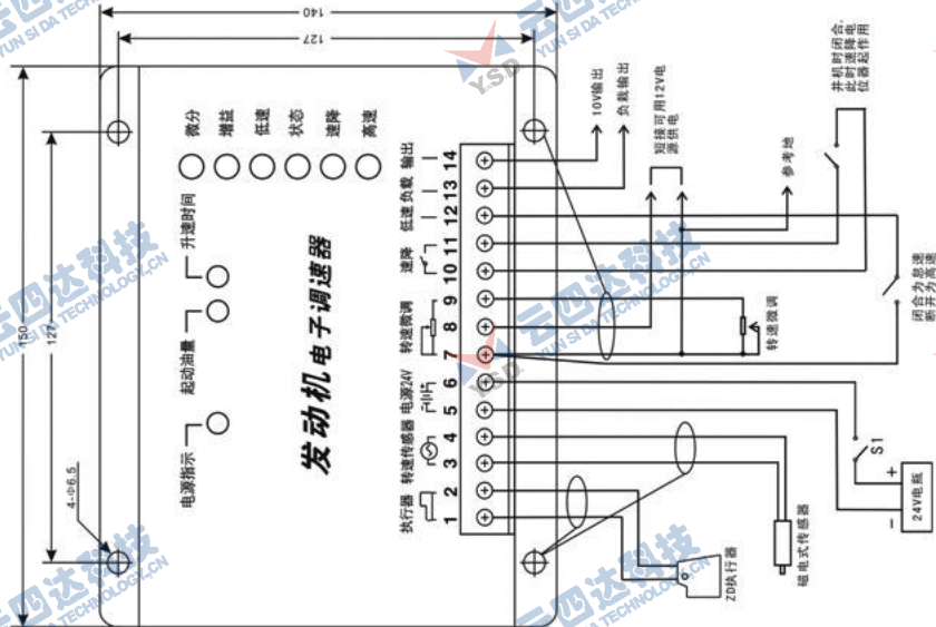
图二. FSK628D控制器用于发电机组安装接线图
