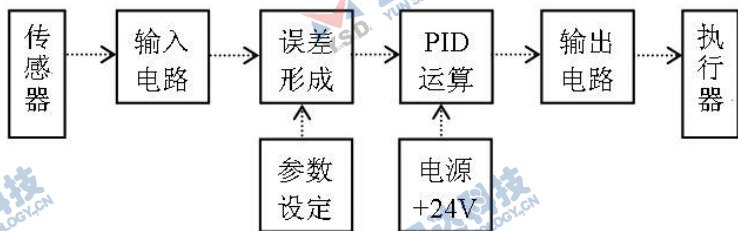
图一、控制器组成
