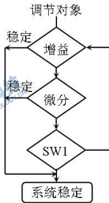
图四. 稳定性调整流程
