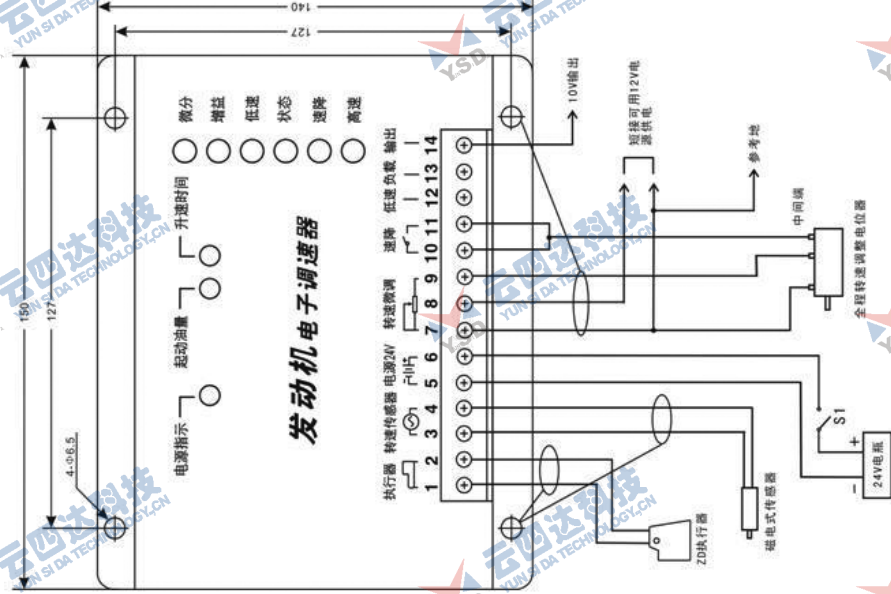
图二. FSK628D控制器用于发电机全程调速接线图
