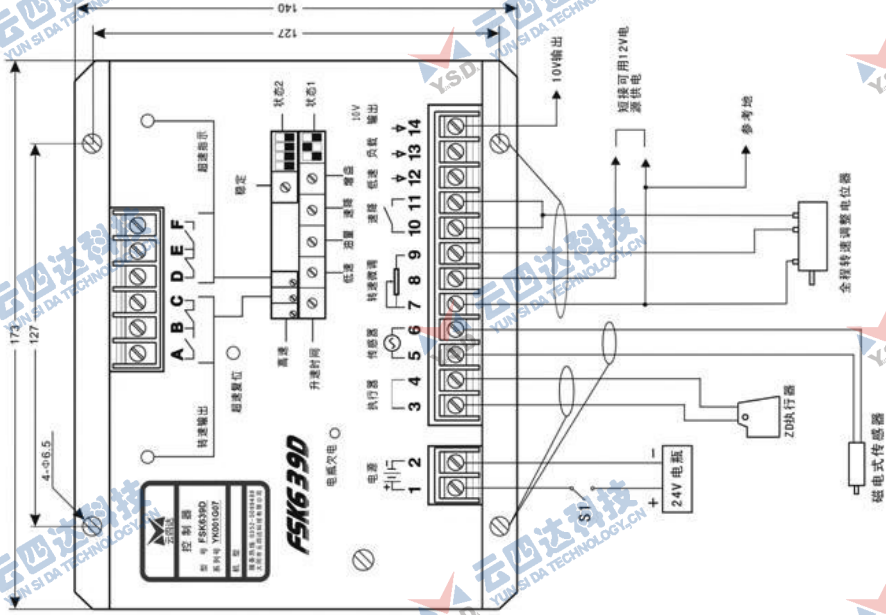
图三.FSK639D 控制器用于发动机全程调速接线图
