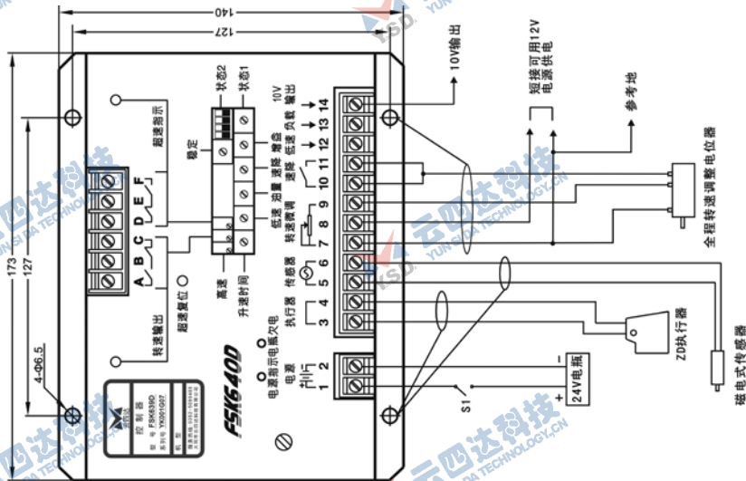
图三: FSK640D控制器用于发电机全程调速接线图
