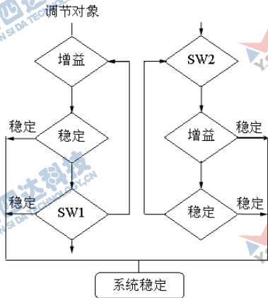
图五. 稳定性调整流程
