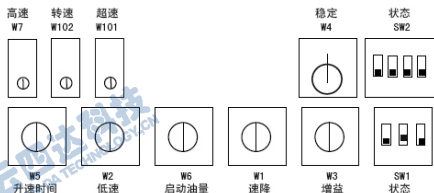
图四 调试窗口示意图
