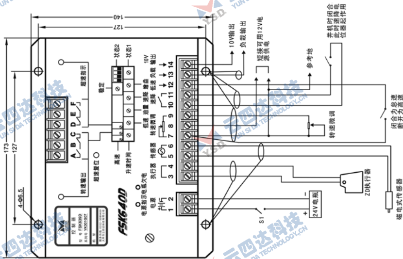
图2. FSK640D控制器用于发电机组安装接线图
