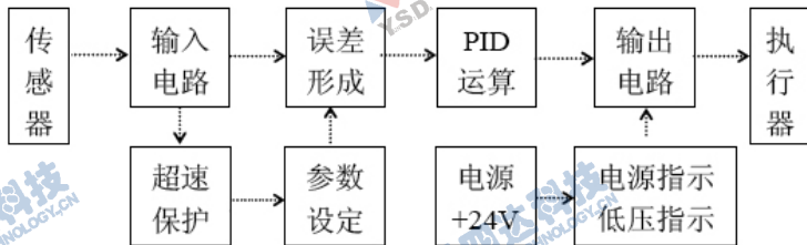
图一、控制器组成
